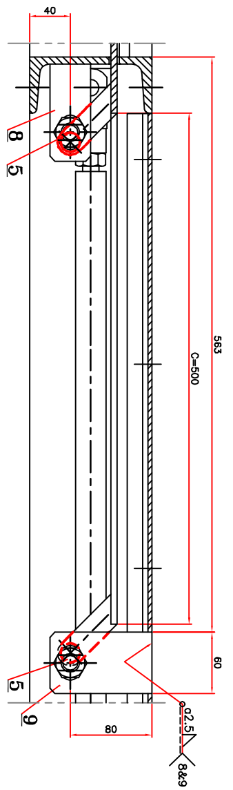
Section E-E Scale: 1:2.5
