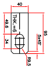
NO 8 Scale: 1:2.5
